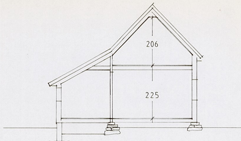
SNITT
