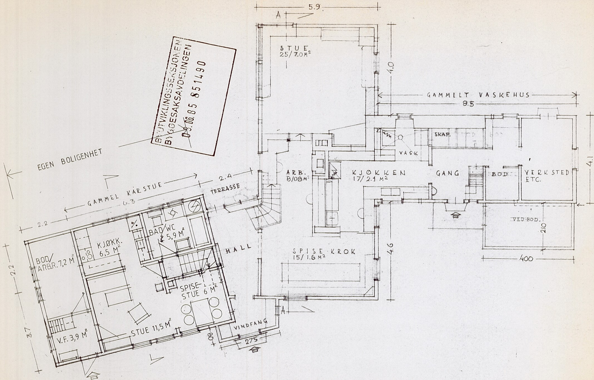
PLAN 1. ETASJE. M 1:100
