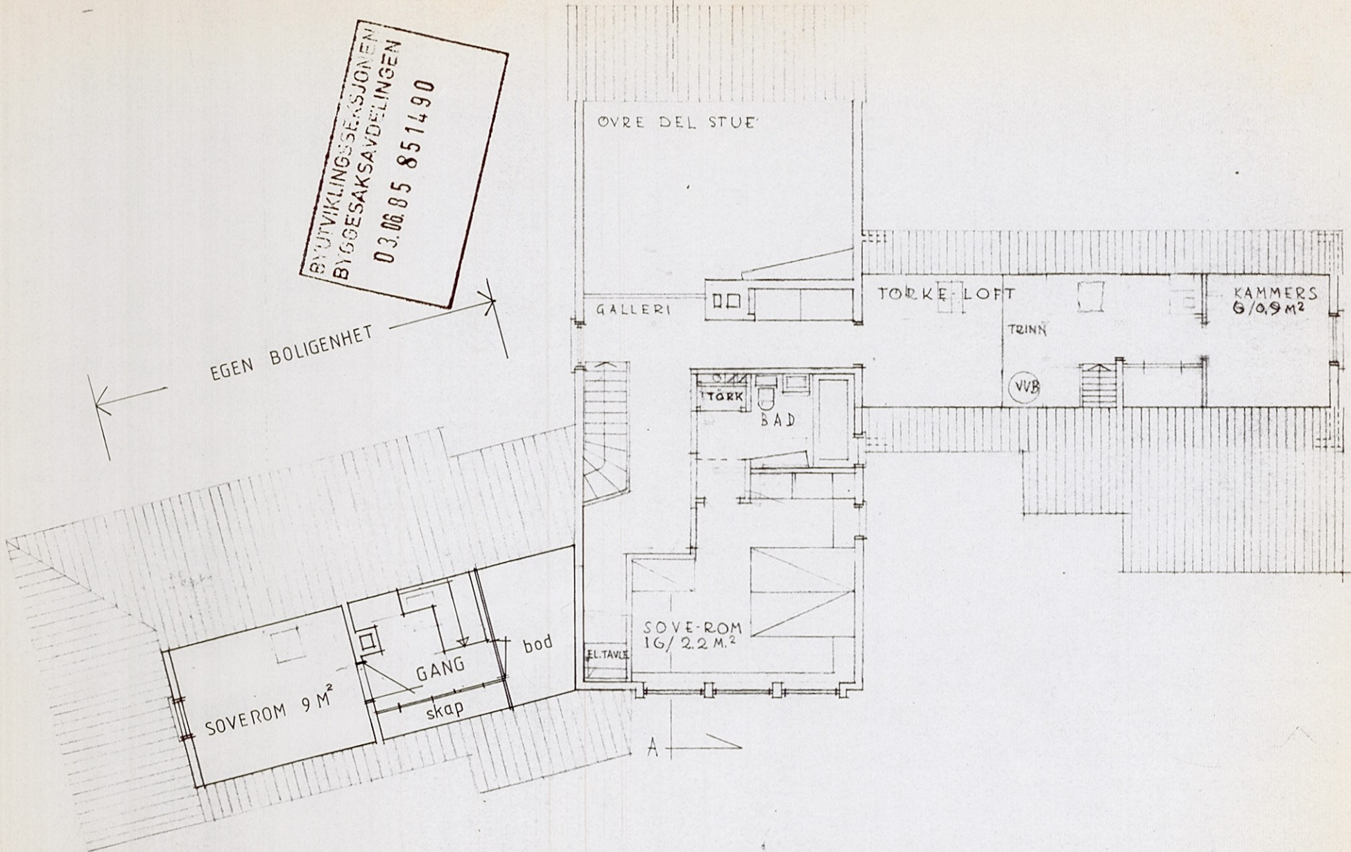
PLAN LOFTS-ETASJE M 1 : 100 ETTER ENDRING.
